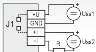
Výstup 4 - 20 mA galvanicky oddělený
