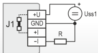
Výstup 4 - 20 mA galvanicky neodělený
