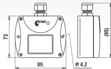
Skříňka s průchodkou
