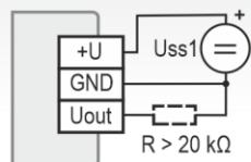
Výstup 0 až 10 V
